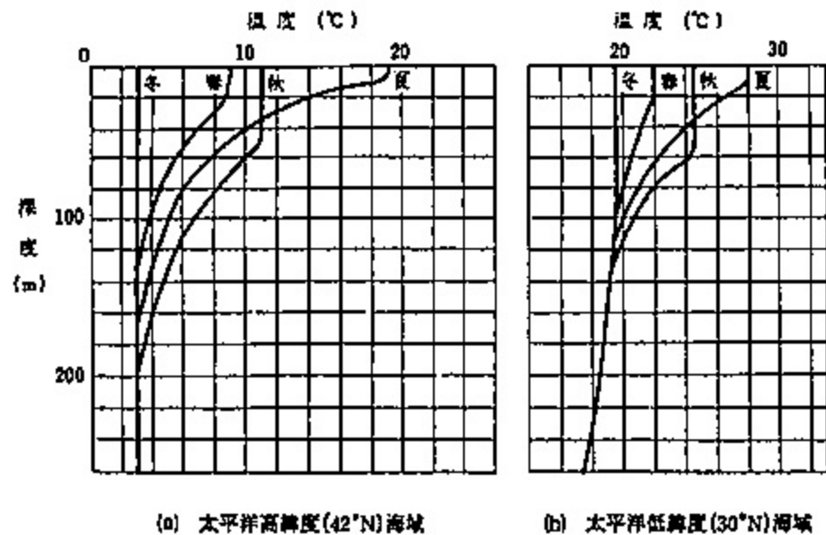
図1. 水温プロファイルの例
